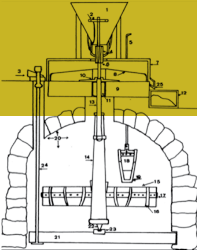
Mecanisme del molí fariner
