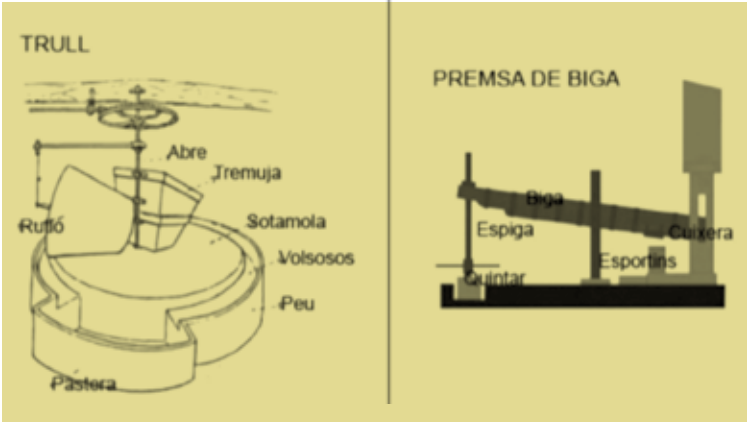
Mecanisme del molí de l'oli
